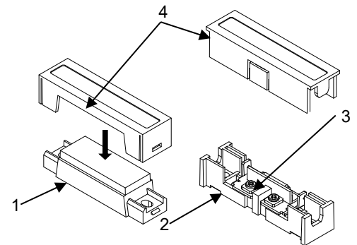
Abbildung 1. Magnetkontakt
